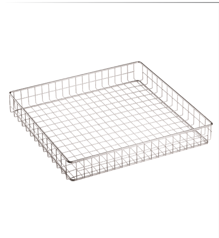
Körbe aus Draht Edelstahl, mit Eckverstärkung Stapelrahmen ø 6 mm Drahtgeflecht ø 2.5 mm Maschenweite 40 x 25 mm • Art. 119745 53x 40 cm h 8.5 cm • Art. 119746 53x40 cm h 12 cm • Art. 119747 53x80 cm h 8.5 cm • Art. 119748 53x80 cm h 12 cm • Art. 119749 50x50 cm h 7.5 cm • Art. 119750 50x50 cm h 11.5 cm
